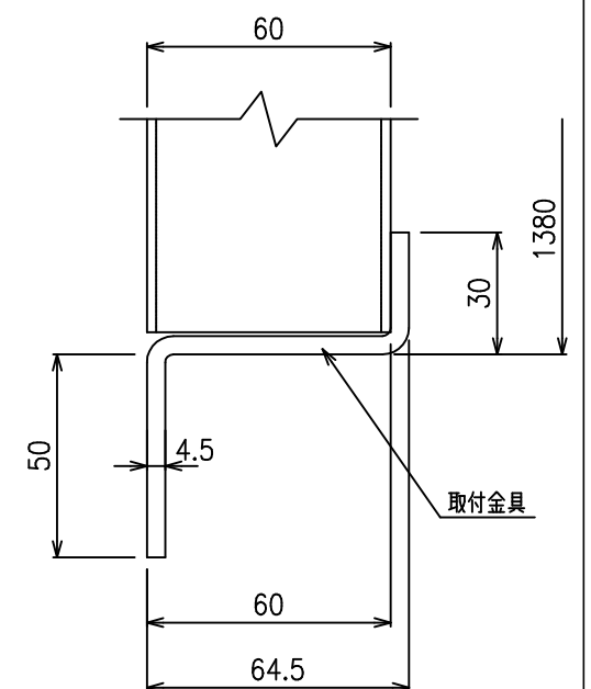
A 詳細図 1/2
