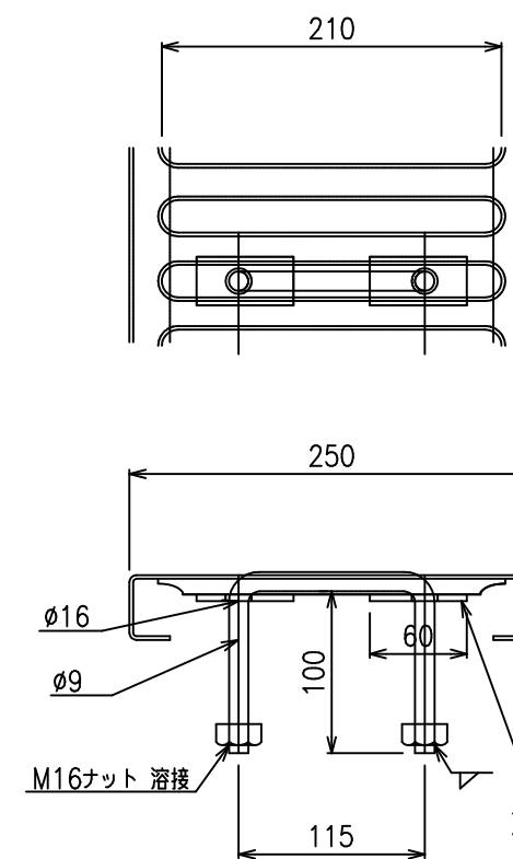
把手詳細図 1/5
