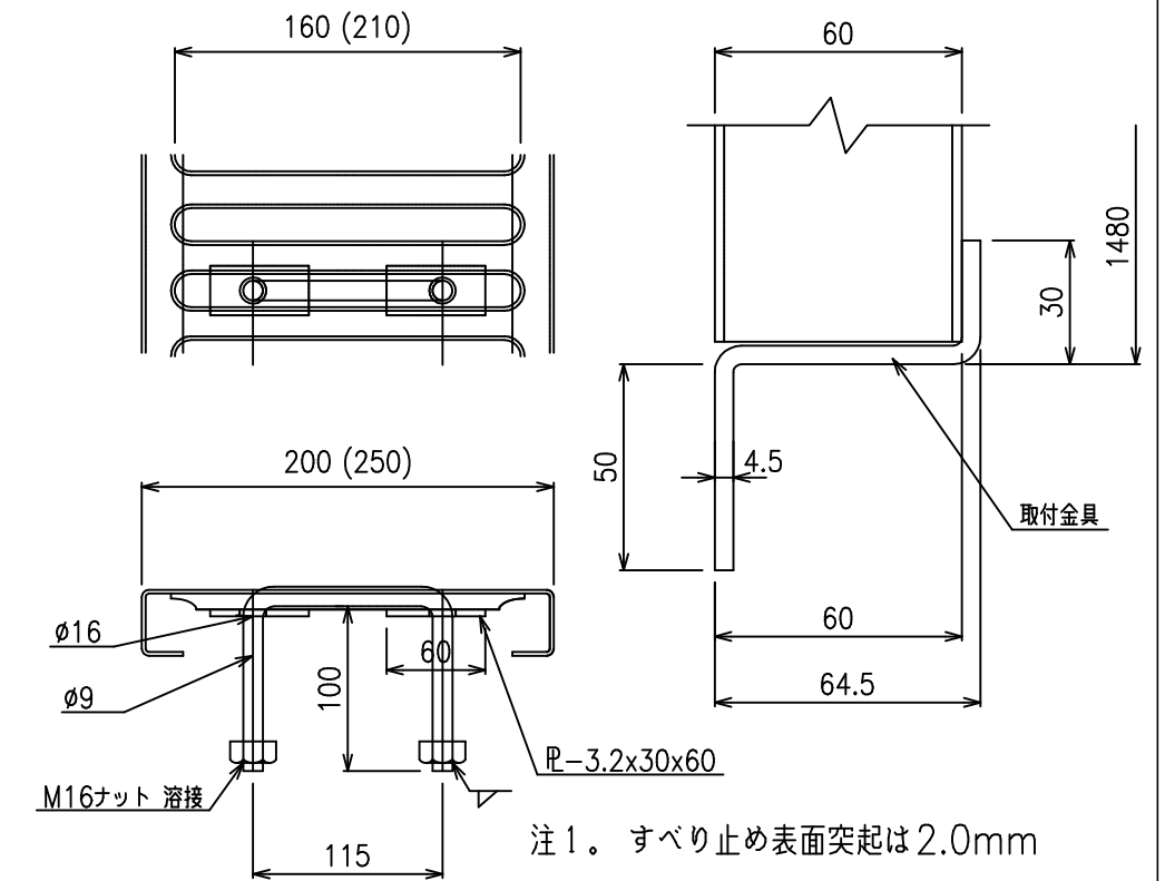
A 詳細図 1/2
