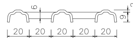
B-B断面
