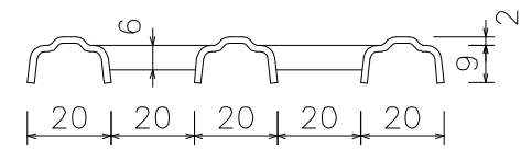
B-B断面
