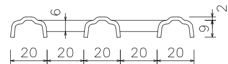
B - B 断面
