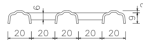
B - B断面
