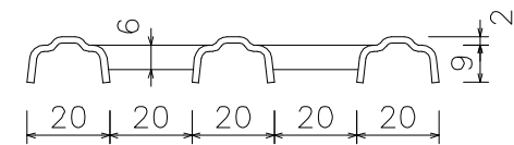
B-B断面
